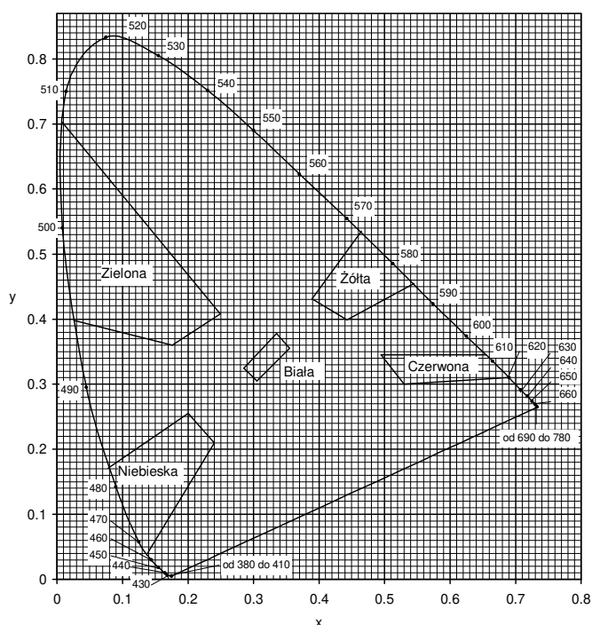
10.33.Rys. 3. Granice barw białej, żółtej, czerwonej, niebieskiej i zielonej oznakowania
