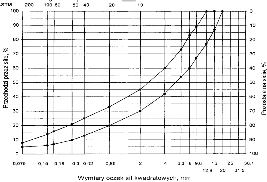
Rys. 7. Krzywe graniczne uziarnienia mieszanki mineralnej BA od 0 do 16 mm do warstwy wyrównawczej i wzmacniającej nawierzchni drogi o obciążeniu ruchem KR3
