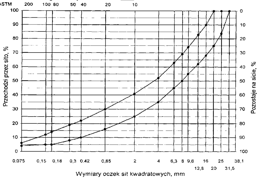
Rys. 6. Krzywe graniczne uziarnienia mieszanki mineralnej BA od 0 do 20 mm do warstwy wyrównawczej i wzmacniającej nawierzchni drogi o obciążeniu ruchem KR3
