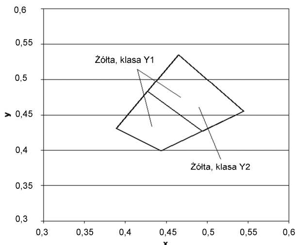
10.32.Rys.2. Współrzędne chromatyczności x,y dla barwy żółtej oznakowania
