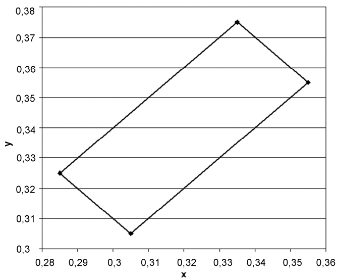
10.31. Rys. 1. Współrzędne chromatyczności x, y dla barwy białej oznakowania
